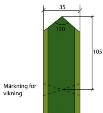
Bild 2.1:7 Vikning av kragspegel m/58. Måttsättning i mm
