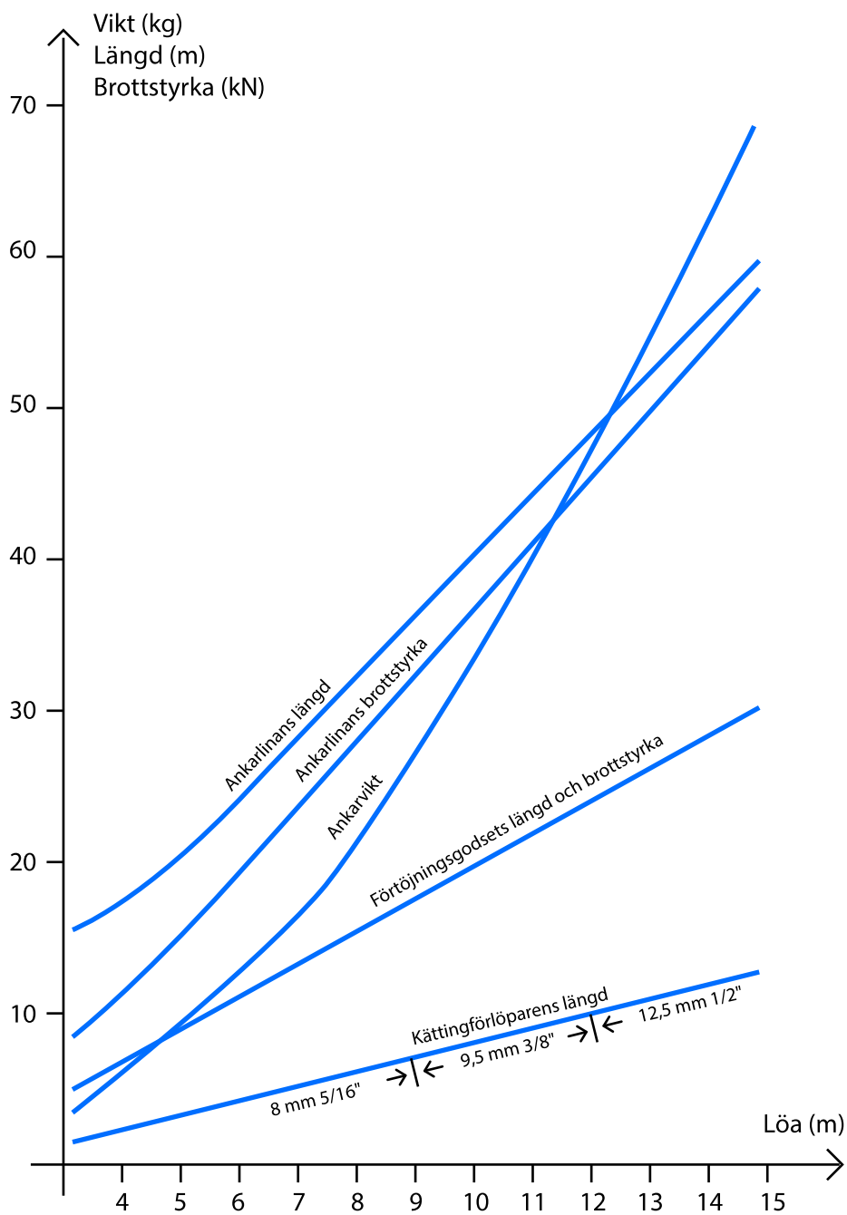
Bild 3:2 Ankrings- och förtöjningsgods för båtar med Löa &lt; 15 m
