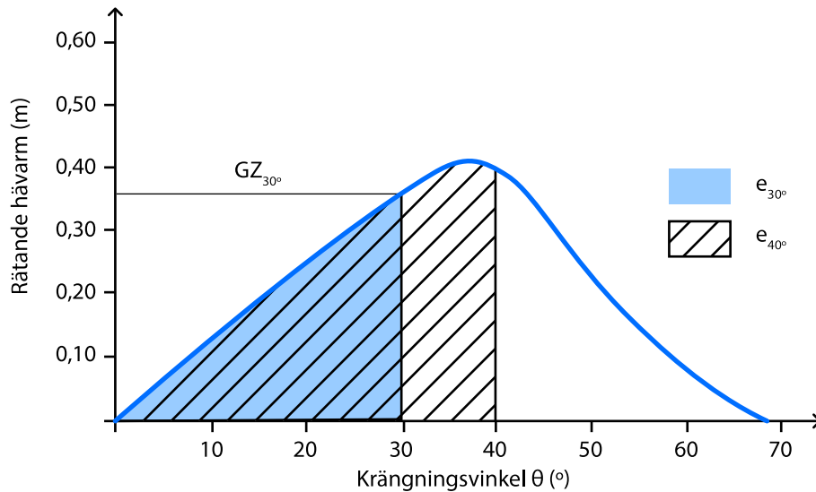
Bild 5:2 GZ-kurva
