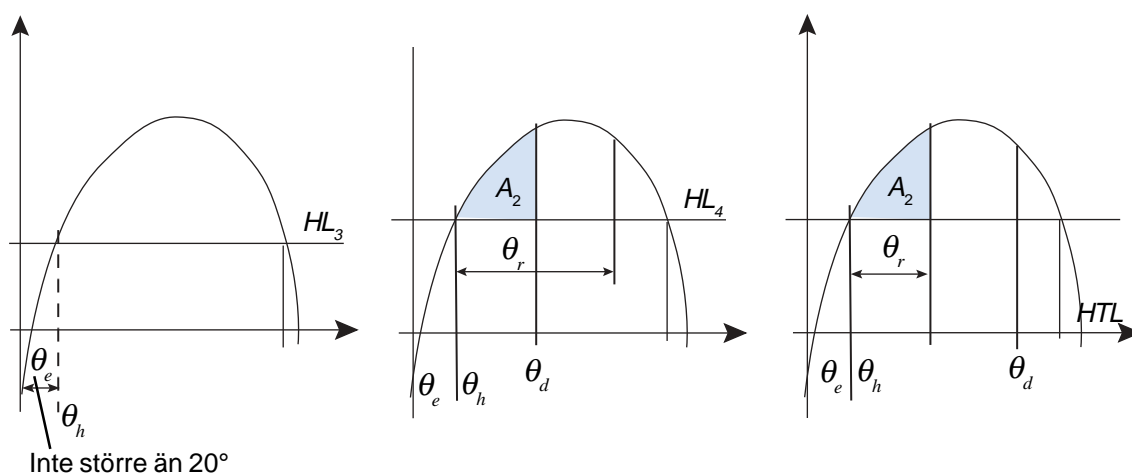
Figur 2. Läckstabilitet.
