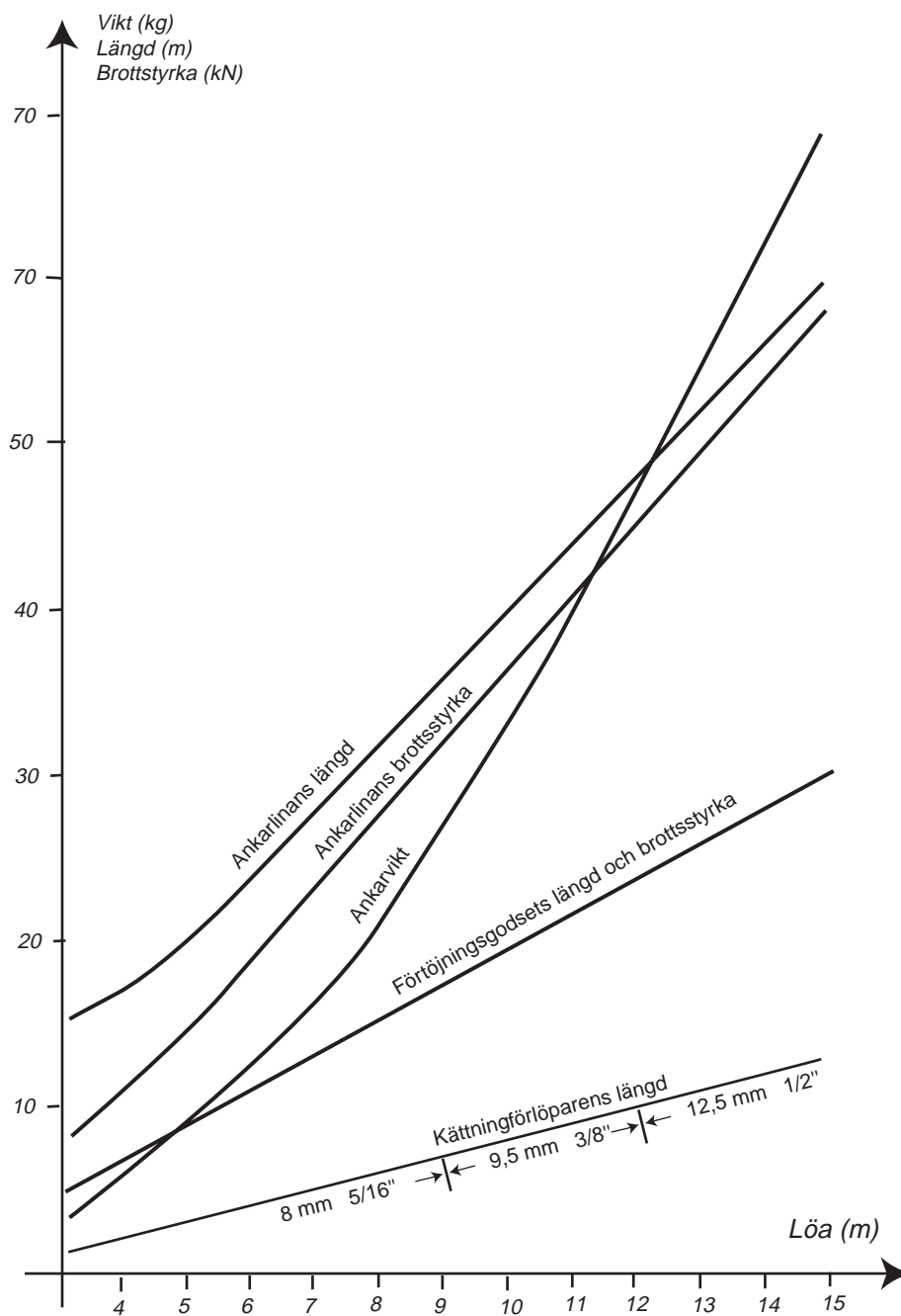
Figur 9.55. Ankrings- och förtöjningsutrustning för båtar med Löt understigande 15 m.
